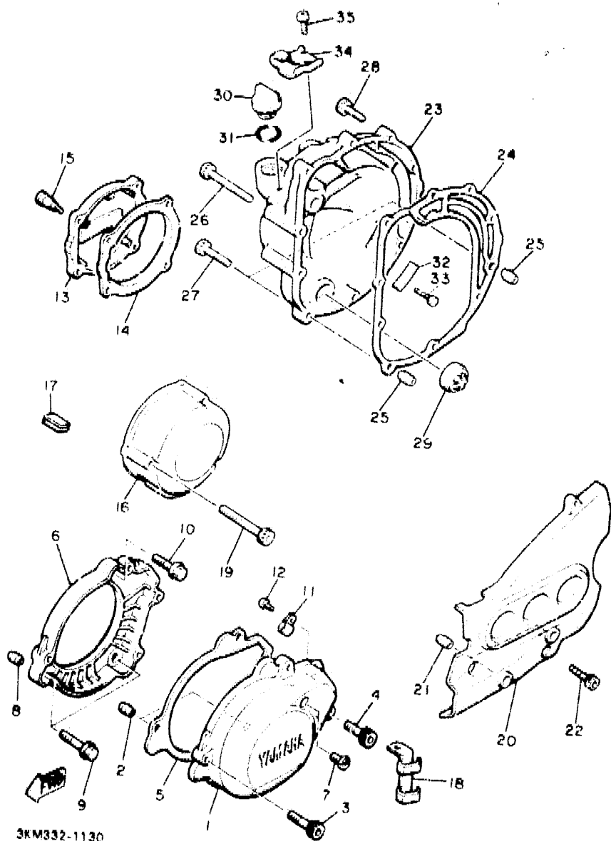
FIG. 13 CUBIERTA DE CARTER 1
