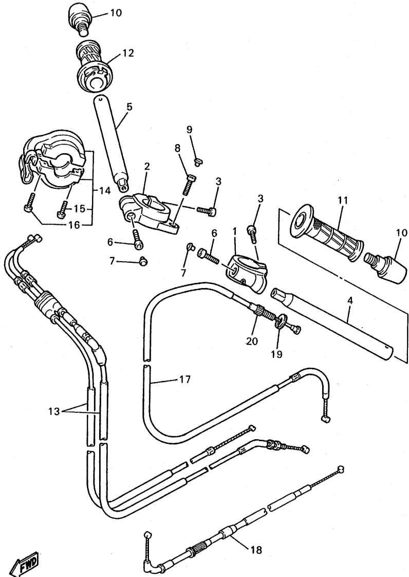
FIG. 33 MANUBRIO. CABLE
