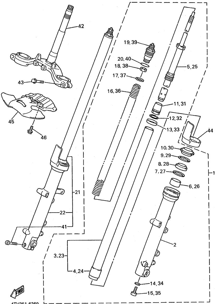
FIG. 26 HORQUILLA DELANTERA
