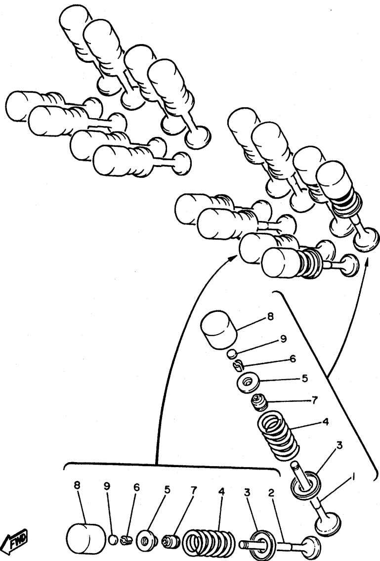
FIG. 4 VALVULA
