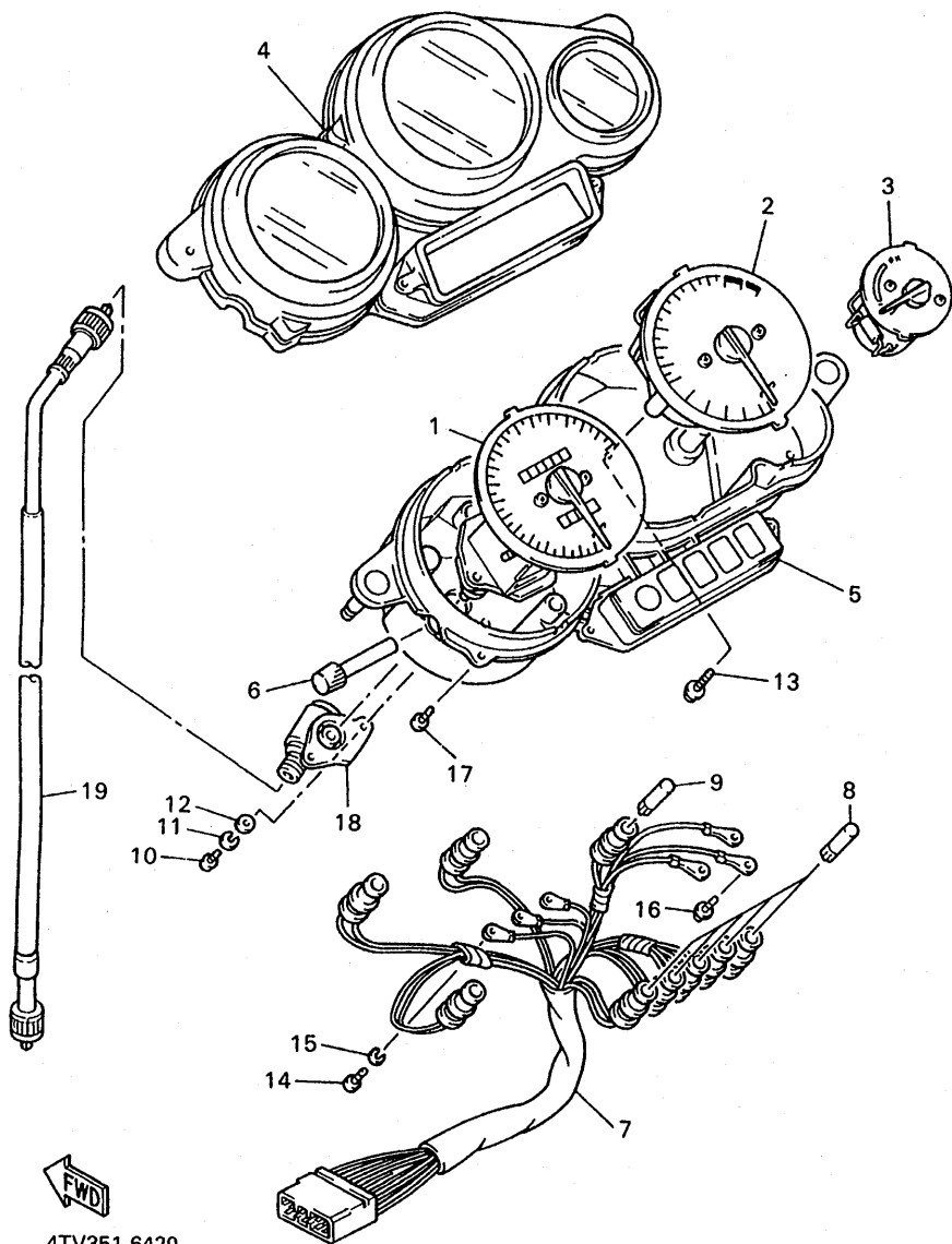
FIG. 42 MEDIDOR
