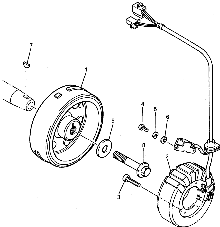
FIG. 39 GENERADOR
