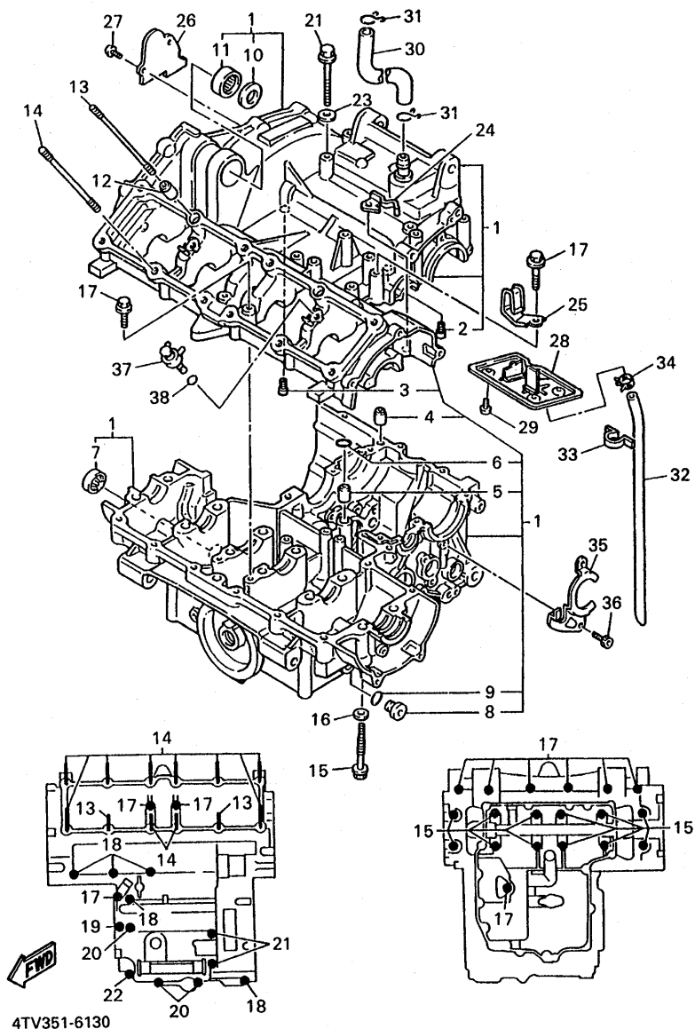
FIG. 13 CARTER
