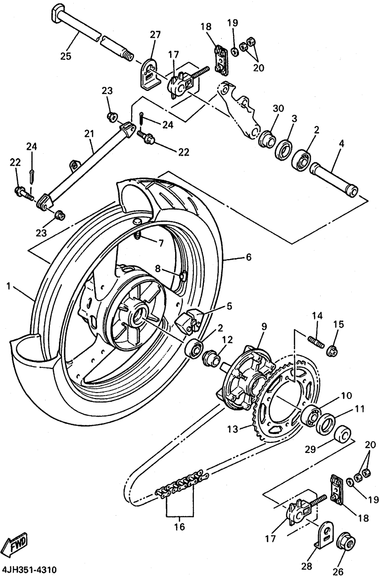
FIG. 31 RUEDA TRASERA
