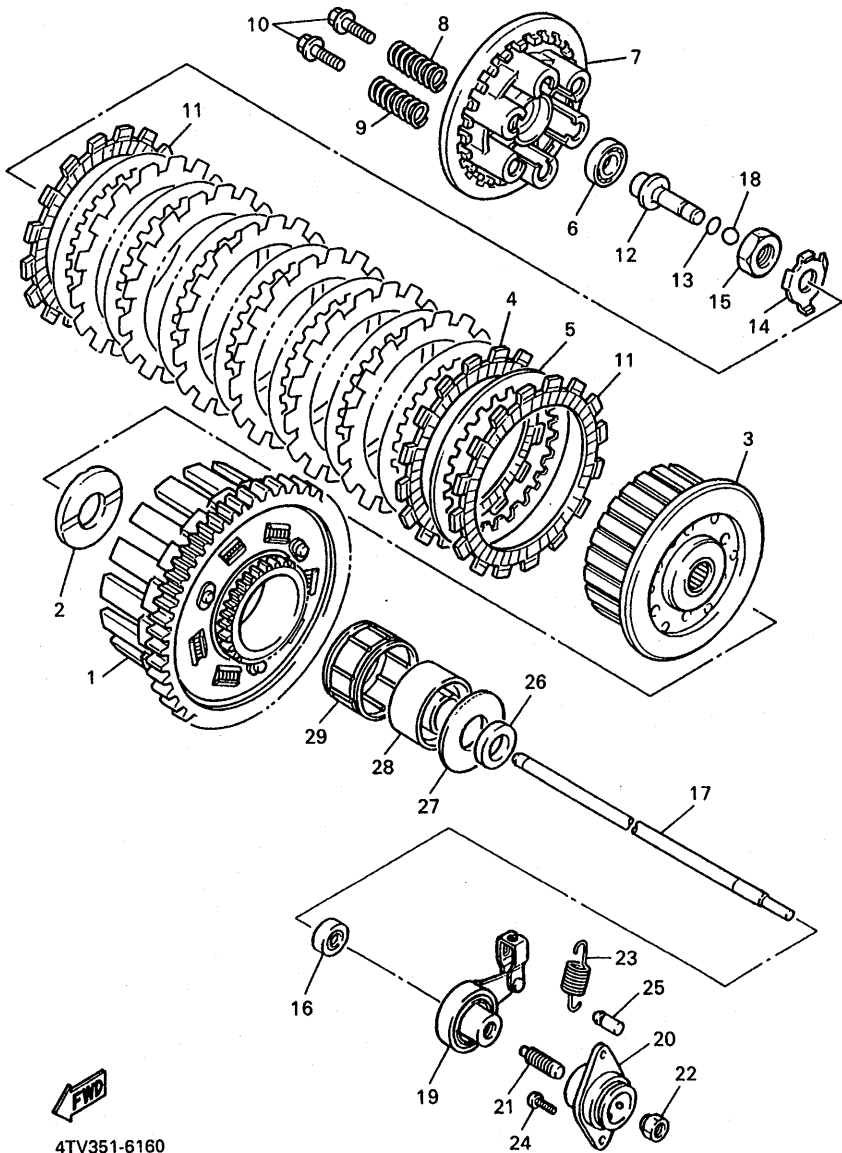
FIG. 16 EMBRAGUE
