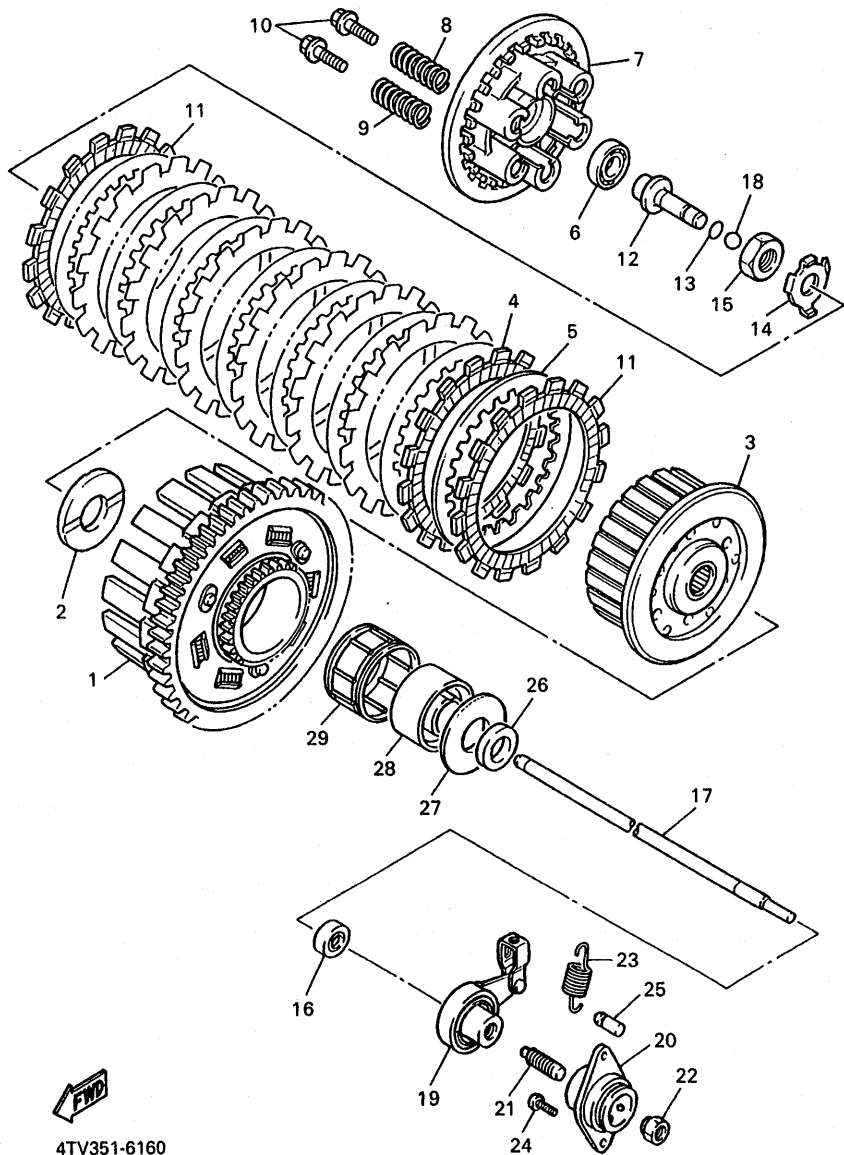
FIG. 16 EMBRAGUE
