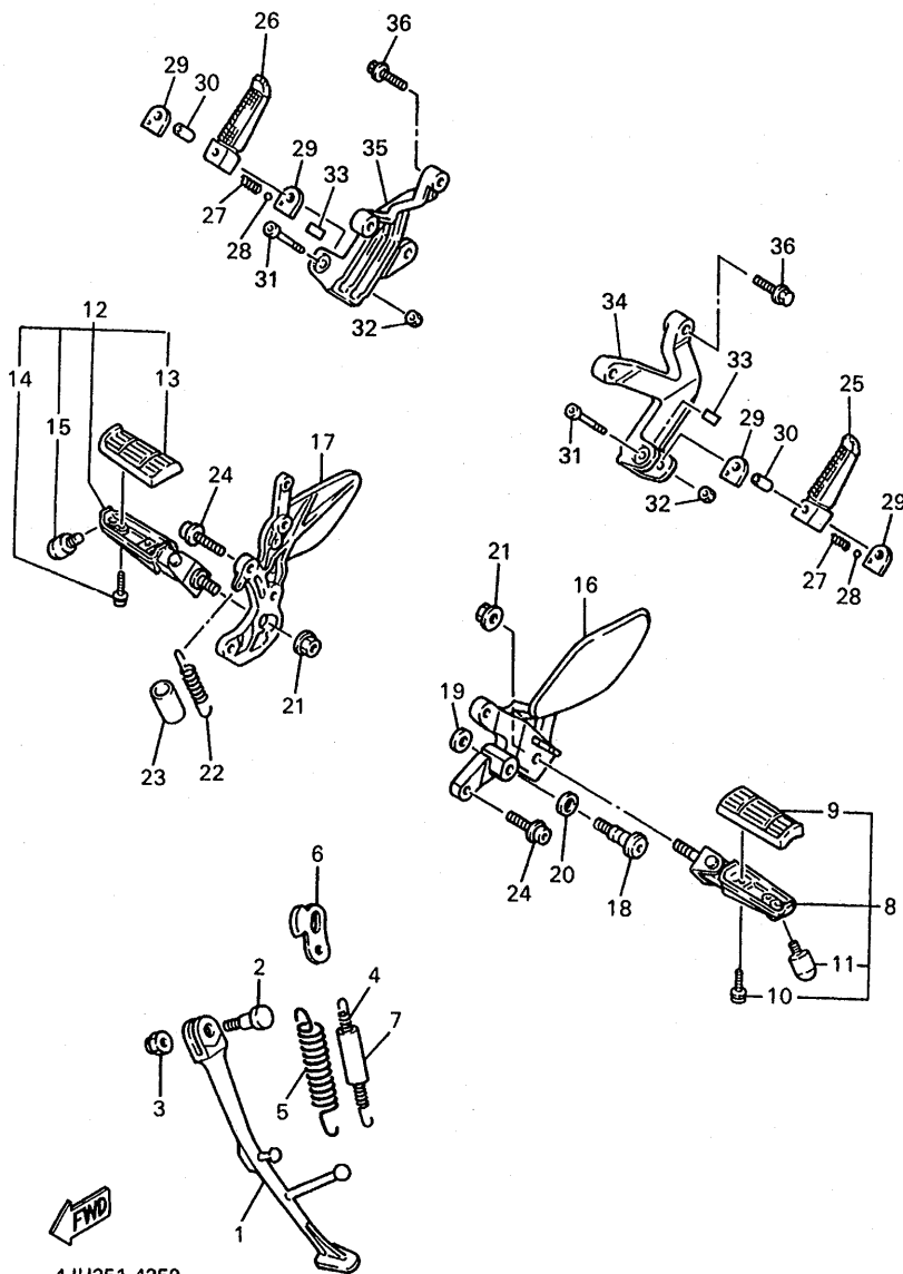
FIG. 35 SOPORTE. APOYAPIE
