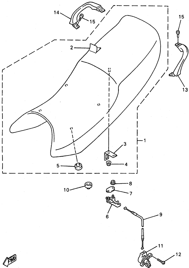
FIG. 28 ASIENTO
