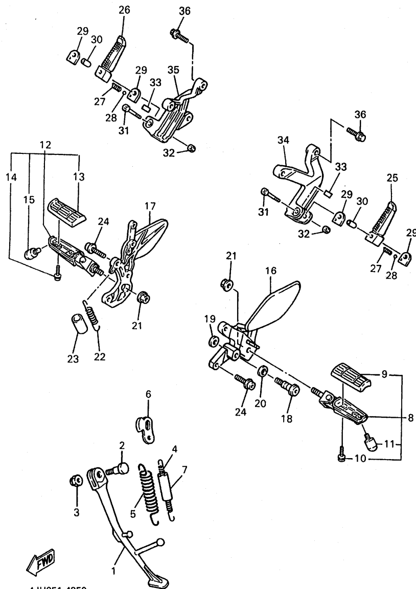
FIG. 35 SOPORTE. APOYAPIE
