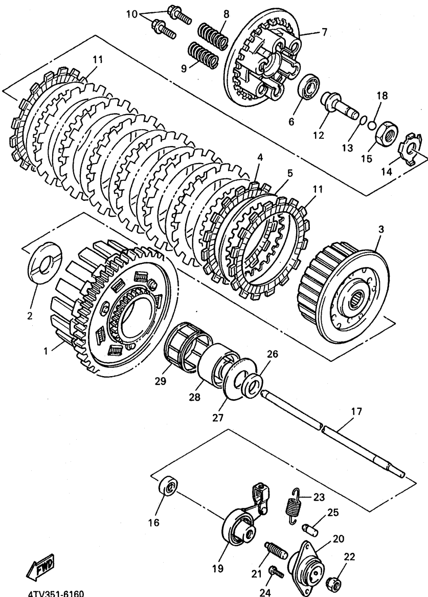
FIG. 16 EMBRAGUE
