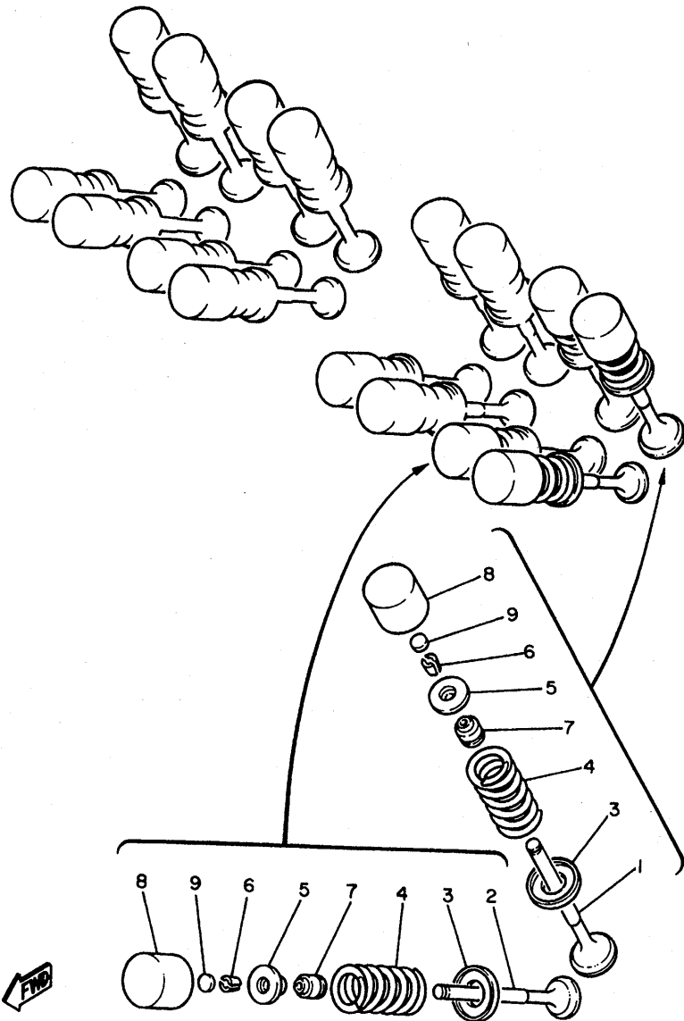
FIG. 4 VALVULA
