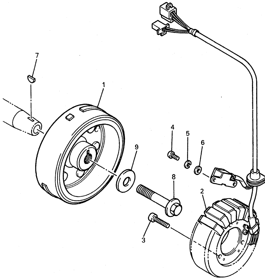
FIG. 39 GENERADOR
