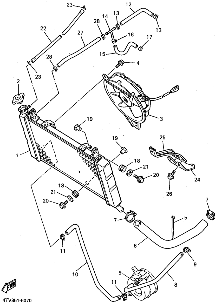
FIG. 7 RADIADOR. MANGUELA
