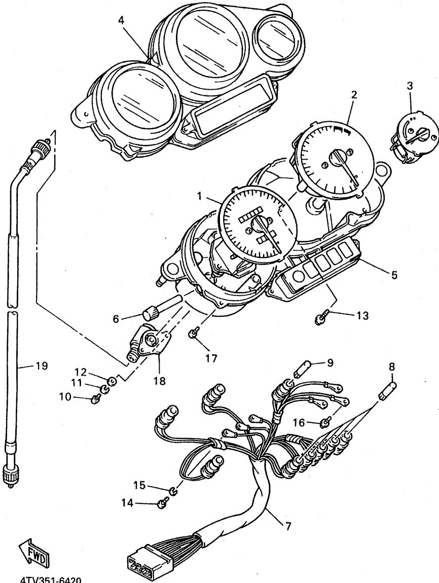
FIG. 42 MEDIDOR
