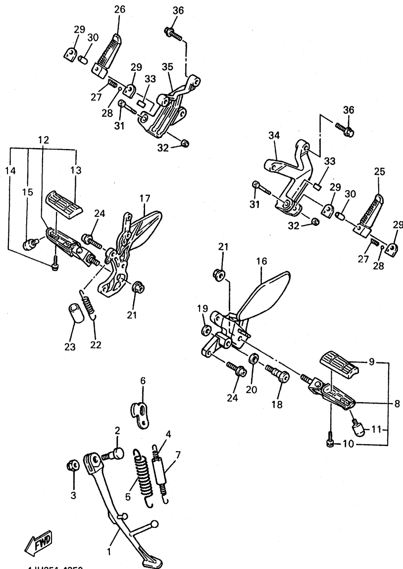
FIG. 35 SOPORTE. APOYAPIE
