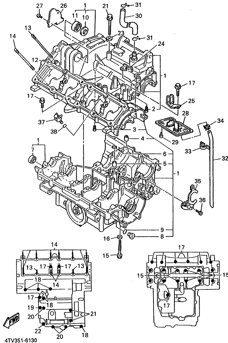
FIG. 13 CARTER
