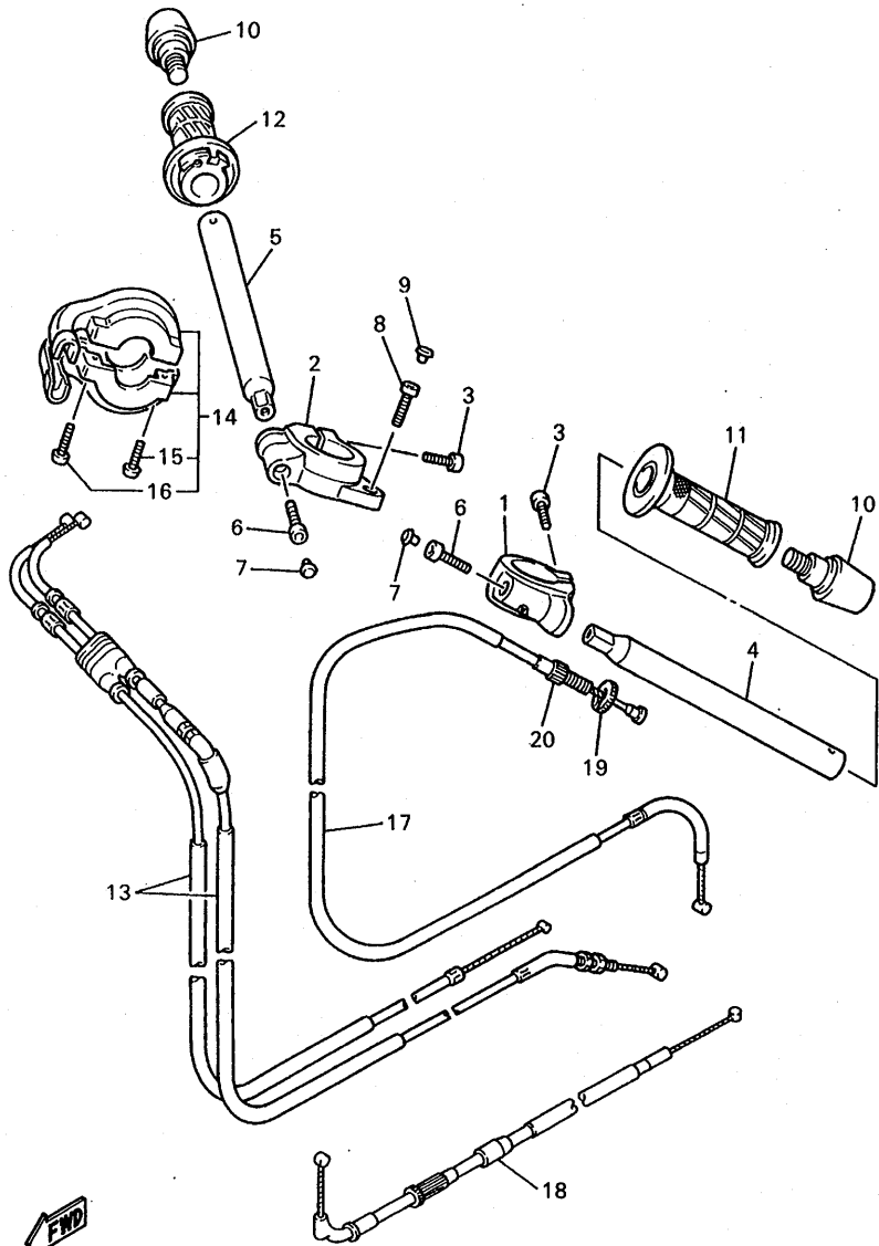
FIG. 33 MANUBRIO. CABLE
