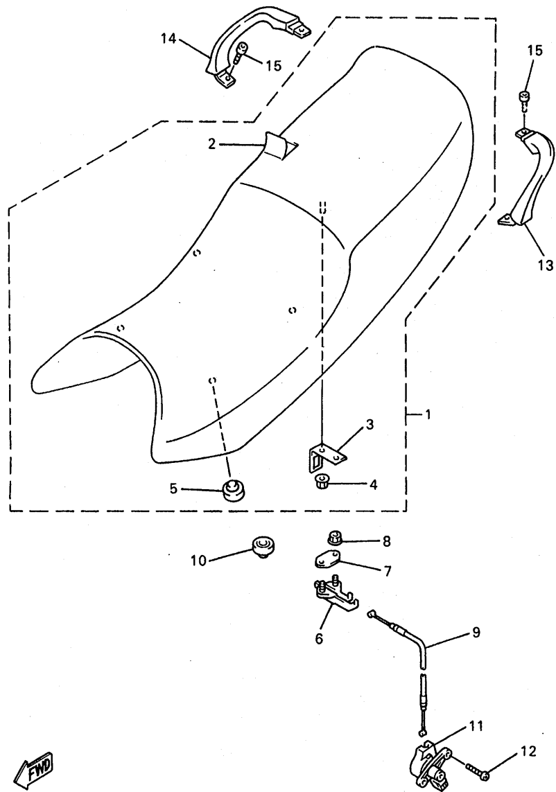
FIG. 28 ASIENTO
