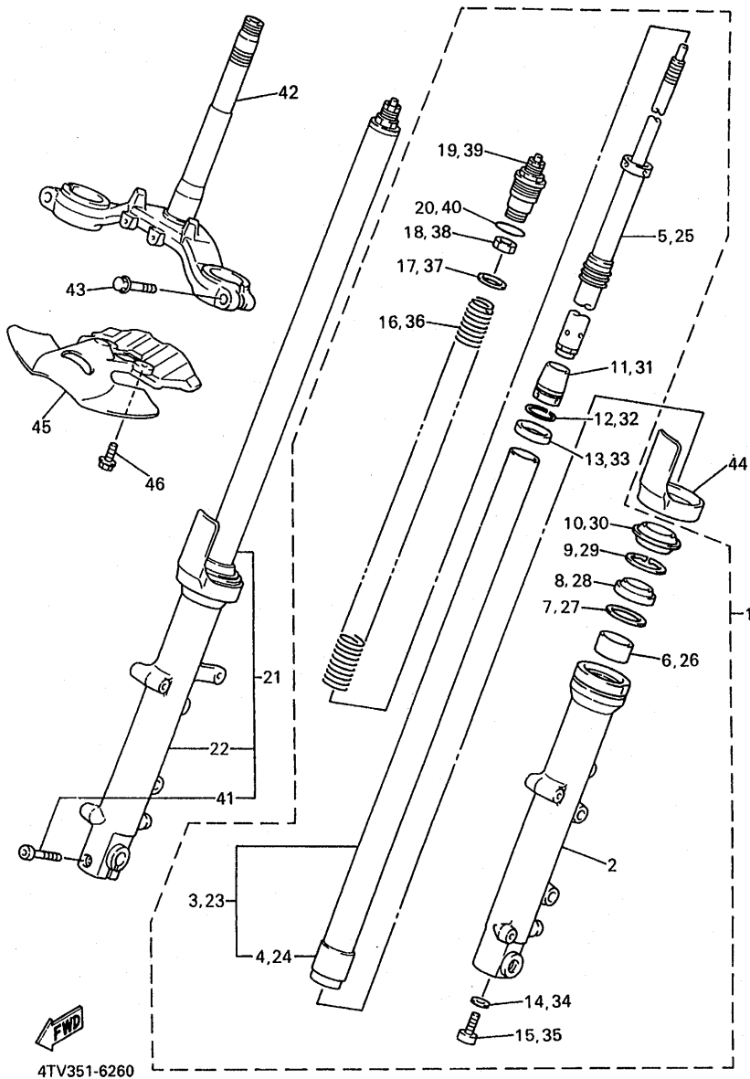
FIG. 26 HORQUILLA DELANTERA
