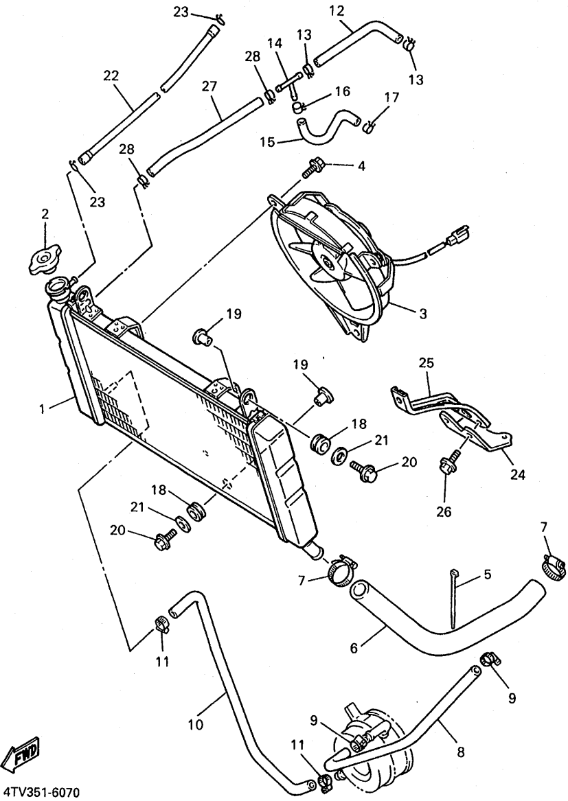
FIG. 7 RADIADOR. MANGUELA
