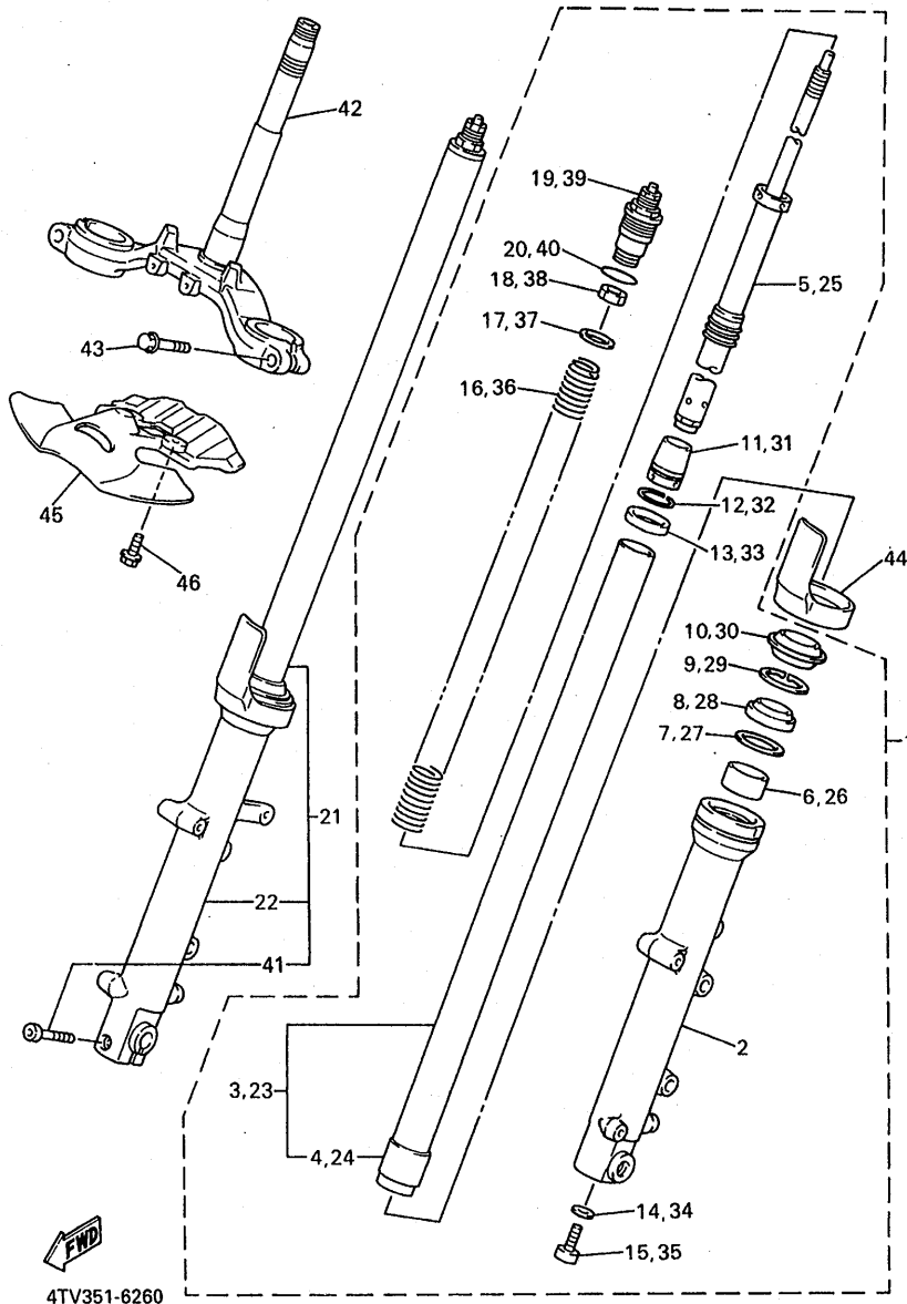
FIG. 26 HORQUILLA DELANTERA
