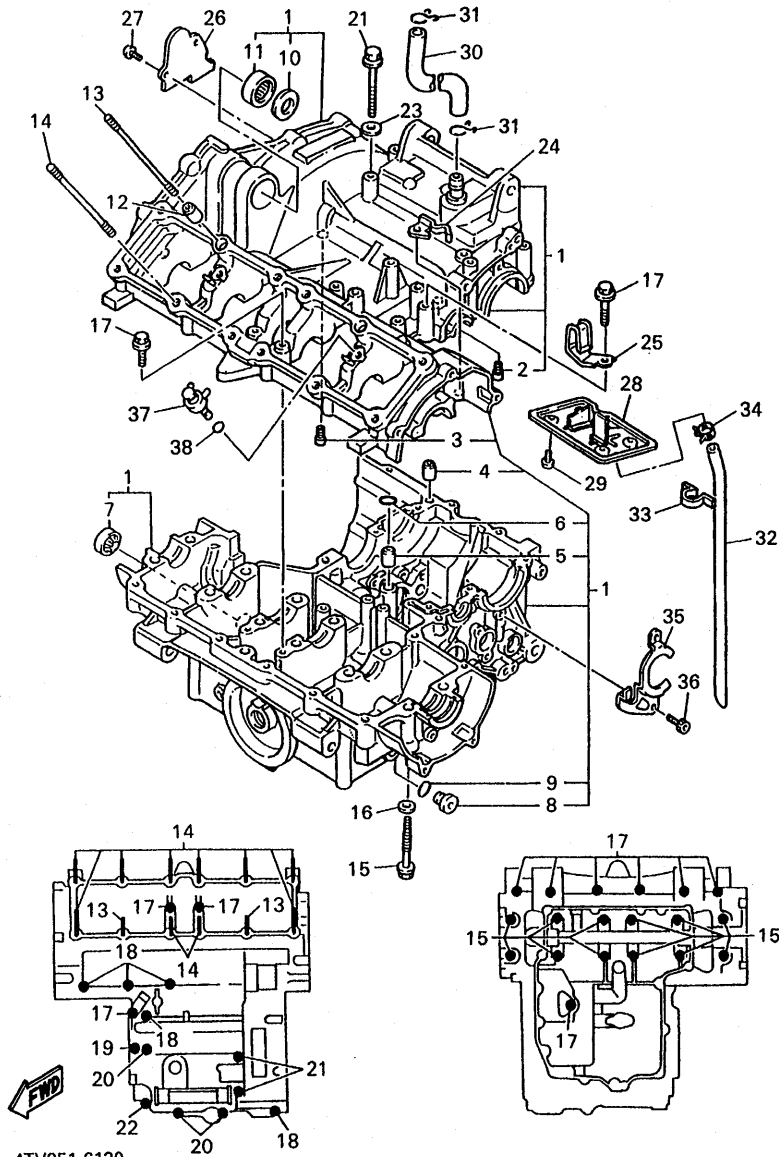
FIG. 13 CARTER
