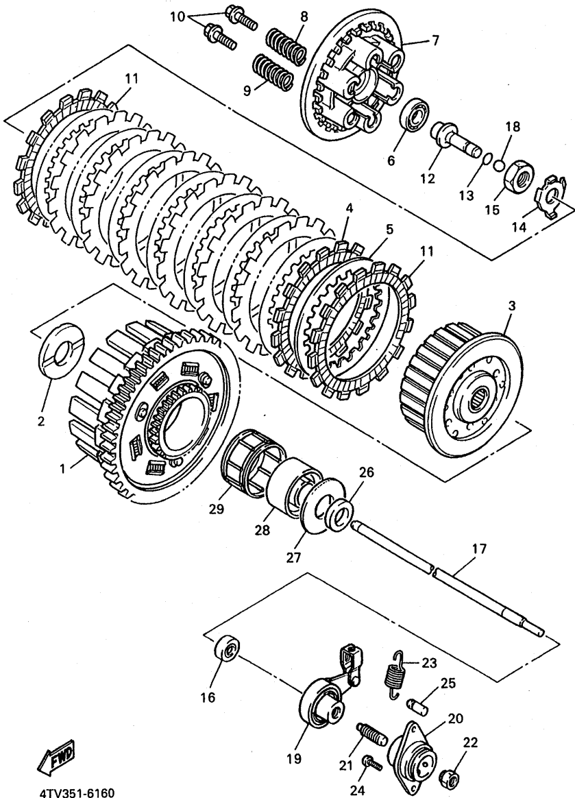
FIG. 16 EMBRAGUE
