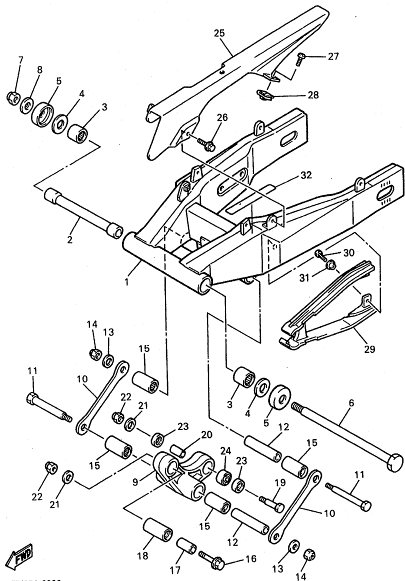
FIG. 23 BRAZO TRASERO
